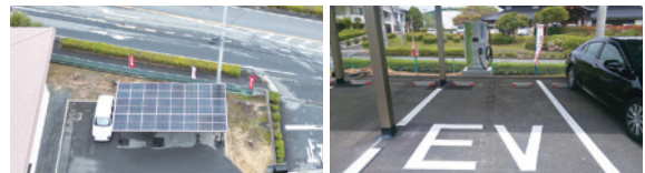
駐車場に設置したソーラーカーポート
